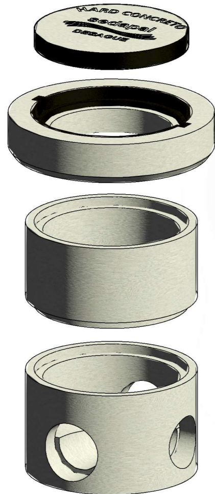
2 COMPONENTES SEPARADOS A103
