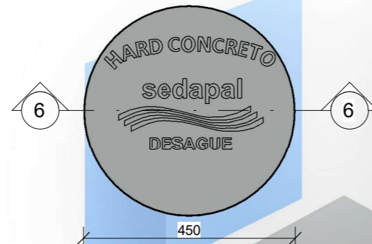
3 TAPA A103 1:10
