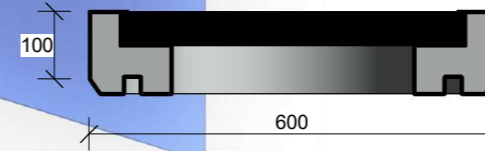
7 7-7 A103 1:10
